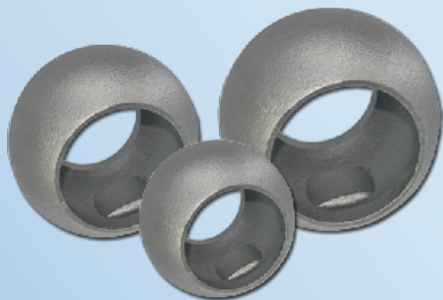
最大毛胚品：不銹鋼鋼球 (直徑 620mm / 內徑 390mm / 高度 471mm / 重量 585.0kg)
