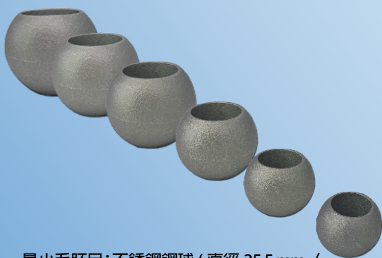
最小毛胚品：不銹鋼鋼球 (直徑 25.5 mm / 內徑 15 mm / 高度 19.6mm / 重量 0.09kg)
